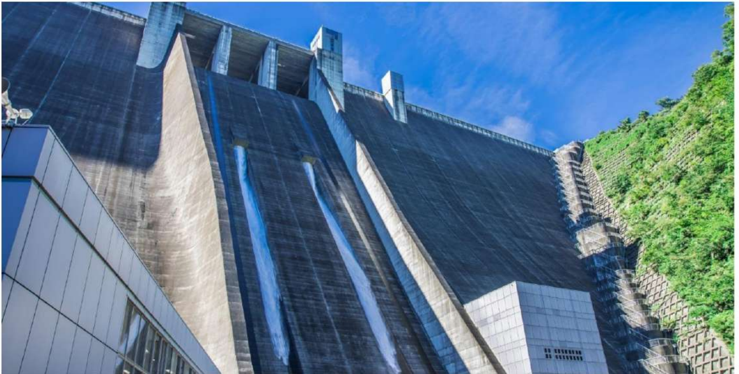
観光放水をしている宮ヶ瀬ダム
